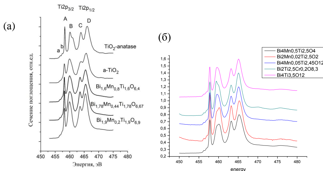
Рис. 5.8. Тонкая структура L_{2,3} Ti2p -спектра поглощения атома титана в аморфном оксиде титана ( \alpha-TiO_2 ), анатазе [158], марганецсодержащих титанатах висмута структурного типа пироклора (а); NEXAFS Ti2p -спектры титанатов висмута структурных типов пироклора и слоистого перовскита (б).
