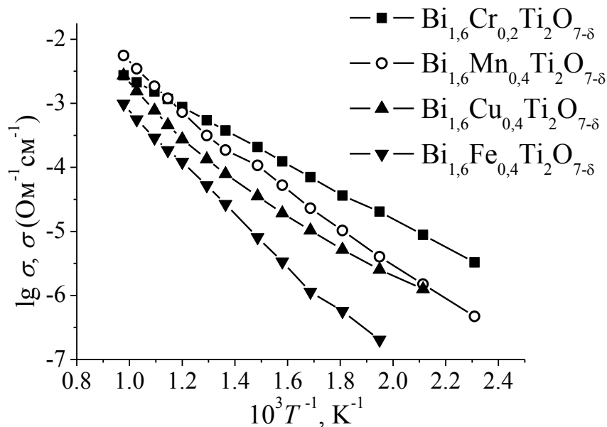
Рис. 7.26. Зависимость проводимости допированных титанатов висмута структурного типа пирохлора от температуры.
