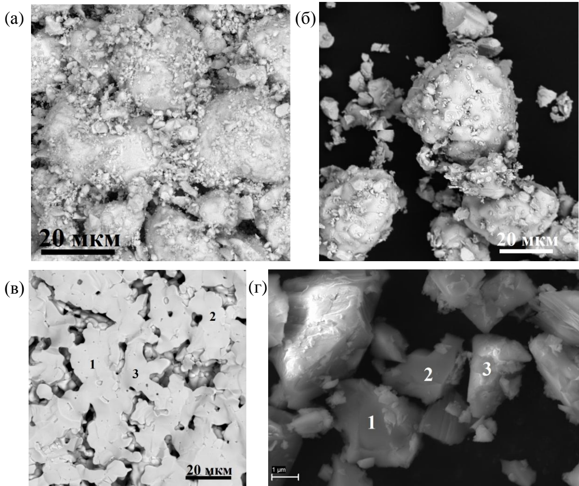
Рис. 3.13. Морфология порошков \text{Bi}_{1,6}\text{Cr}_{0,16}\text{Ti}_2\text{O}_{7-\delta} (а), \text{Bi}_{1,55}\text{Cu}_{0,61}\text{Ti}_2\text{O}_{7-\delta} (б), \text{Bi}_2\text{Mn}_{0,3}\text{Ti}_2\text{O}_{7-\delta} ( \text{Bi}_{1,86}\text{Mn}_{0,29}\text{Ti}_{1,86}\text{O}_{7-\delta} ) (в); \text{Bi}_2\text{Mn}_1\text{Ti}_2\text{O}_{7-\delta} ( \text{Bi}_{1,6}\text{Mn}_{0,8}\text{Ti}_{1,6}\text{O}_{7-\delta} ) (г) (твердофазный метод получения, 1050 °С).
