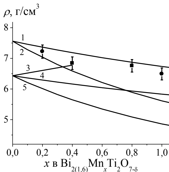
Рис. 4.7. Пикнометрические и рентгенографические плотности марганецсодержащих титанатов висмута, для разных моделей распределения атомов марганца по позициям структуры пирохлора ( a = 10,321 \text{ \AA} ).
