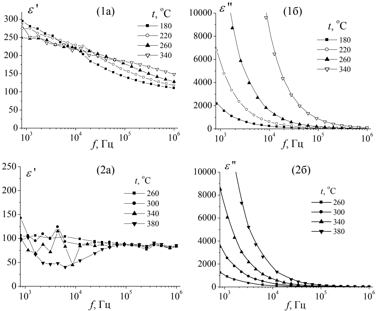
Рис. 7.17. Частотные зависимости действительной \varepsilon' (а) и мнимой \varepsilon'' (б) части диэлектрической проницаемости \text{Bi}_{1,6}\text{Mn}_{0,8}\text{Ti}_{1,6}\text{O}_{7-\delta} (1а,1б) и \text{Bi}_{1,86}\text{Mn}_{0,28}\text{Ti}_{1,86}\text{O}_{7-\delta} (2а,2б) при разных температурах.
