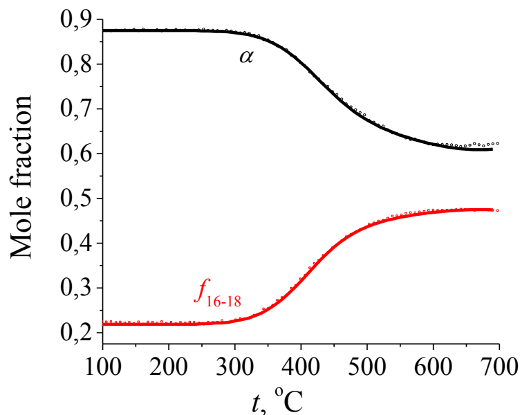
Рис. 7.28. Зависимости атомной доли ( \alpha^{18} ) ^{18}\text{O} в газофазном кислороде от температуры в проточном реакторе.
