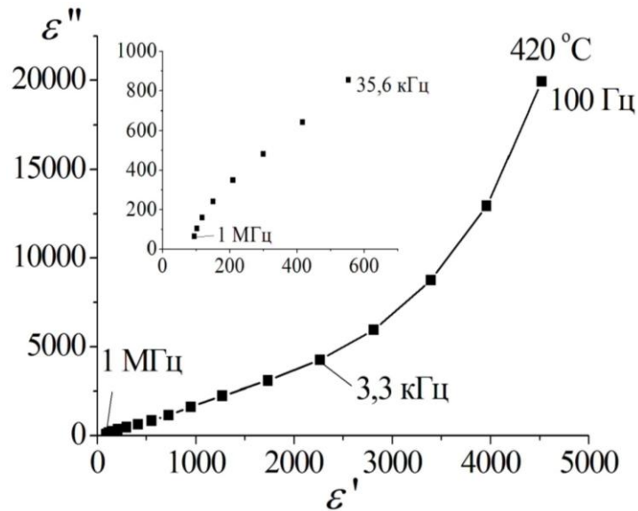
Рис. Г.4. Зависимости \varepsilon''(\varepsilon') \text{Bi}_{1,6}\text{Fe}_{0,30}\text{Ti}_2\text{O}_{7-\delta} при 420^\circ\text{C} .
