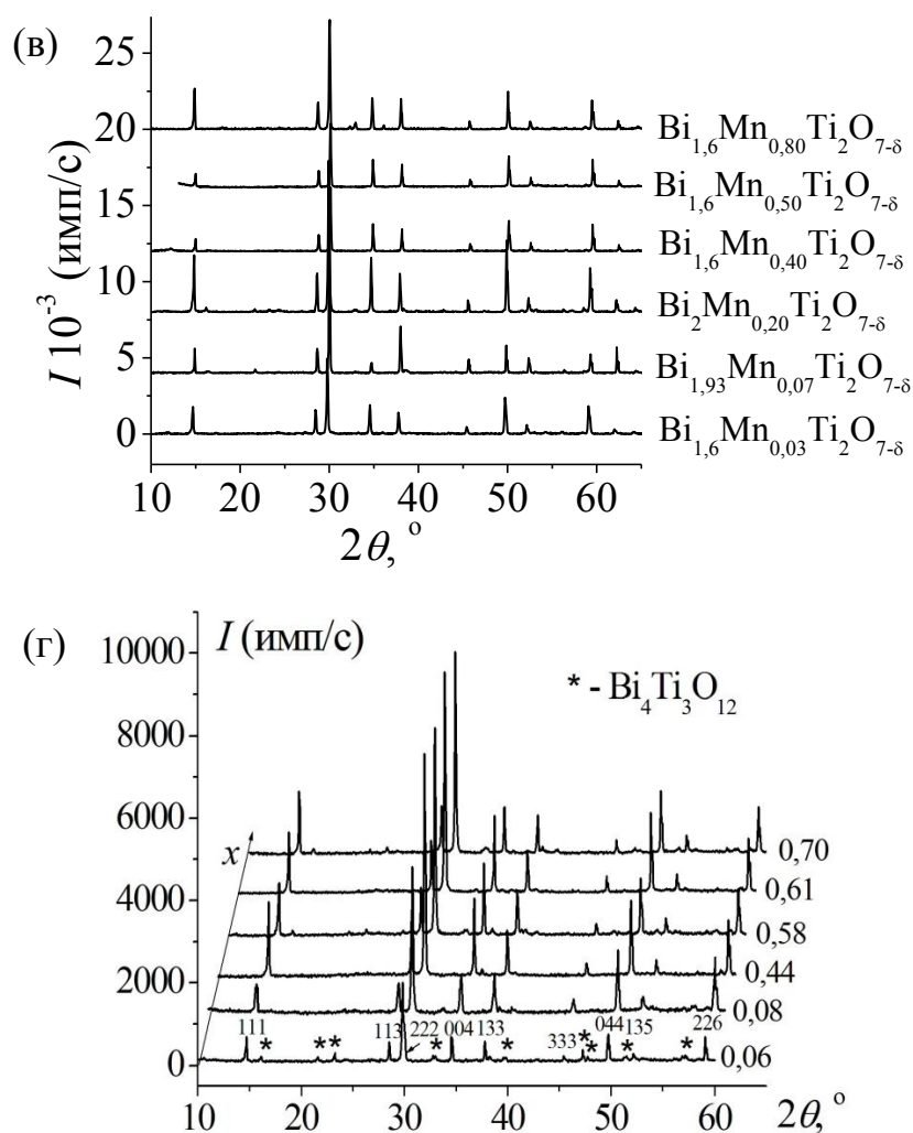
Рис. 3.2. Дифрактограммы \text{Bi}_{1,6}\text{M}_x\text{Ti}_2\text{O}_{7-\delta} структурного типа пироклора ( M - \text{Cr} (а), \text{Fe} (б), \text{Mn} (в), \text{Cu} (г)).
