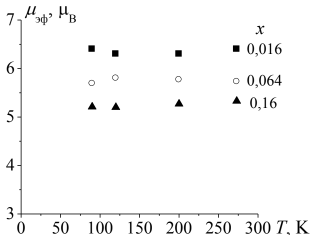
Рис. 6.9. Магнитный момент для \text{Bi}_2\text{Mn}_x\text{Ti}_2\text{O}_{7-\delta} ( \text{Bi}_{1,99}\text{Mn}_{0,0159}\text{Ti}_{1,99}\text{O}_{7-\delta} ; \text{Bi}_{1,97}\text{Mn}_{0,063}\text{Ti}_{1,97}\text{O}_{7-\delta} ; \text{Bi}_{1,92}\text{Mn}_{0,15}\text{Ti}_{1,92}\text{O}_{7-\delta} ).
