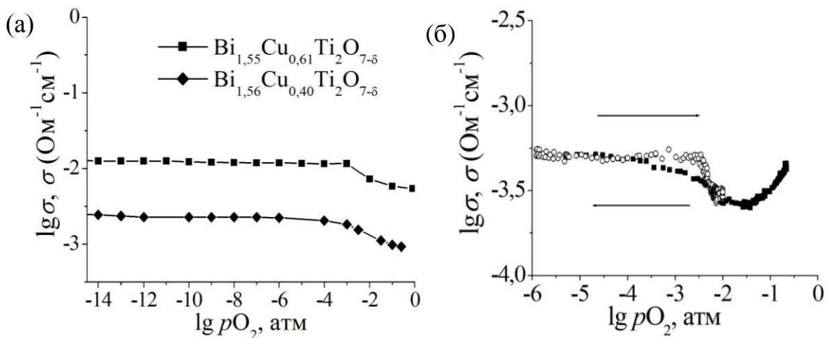
Рис. 7.27. Зависимость проводимости медь- и железосодержащих титанатов висмута \text{Bi}_{1,6}\text{Cu}_x\text{Ti}_2\text{O}_{7-\delta} (а) и \text{Bi}_{1,6}\text{Fe}_{0,42}\text{Ti}_2\text{O}_{7-\delta} (б) от парциального давления кислорода \lg p(\text{O}_2) при 750 °С (стрелками показаны режимы уменьшения и увеличения давления кислорода).
