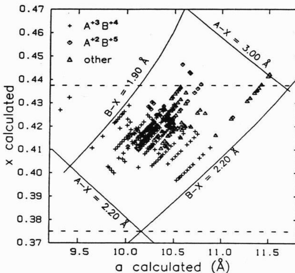
Рис. 1.8. Рассчитанные параметры элементарной ячейки и позиционный параметр x аниона в аппроксимированном диапазоне образования пироклора A_2B_2X_6Y . Сплошные линии показывают величины длин связей в кубическом и октаэдрическом полиэдрах [75].
