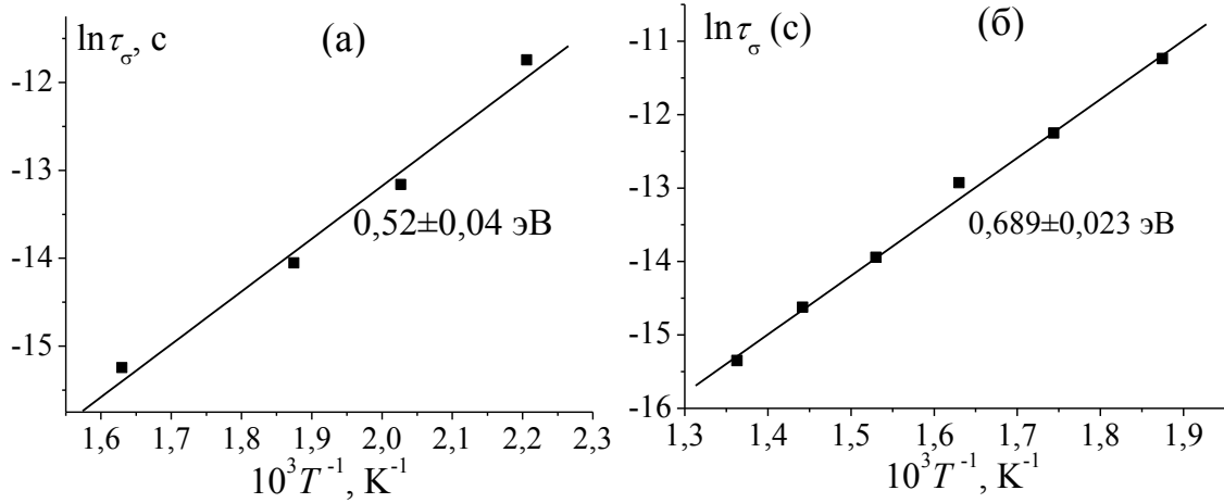
Рис. 7.19 Зависимость логарифма времени релаксации \tau_{\sigma} (с) от обратной температуры для \text{Bi}_{1,6}\text{Mn}_{0,8}\text{Ti}_{1,6}\text{O}_{7-\delta} (а) и \text{Bi}_{1,86}\text{Mn}_{0,28}\text{Ti}_{1,86}\text{O}_{7-\delta} (б).
