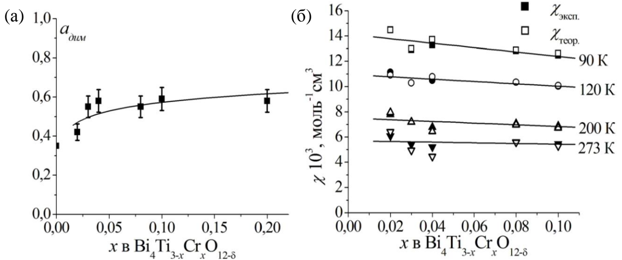
Рис. 6.2. Доли димеров хрома a_2 в \text{Bi}_4\text{Ti}_{3-x}\text{Cr}_x\text{O}_{12-\delta} (а); расчетные (светлые значки) величины магнитной восприимчивости и ее экспериментальные значения (темные значки) (б).
