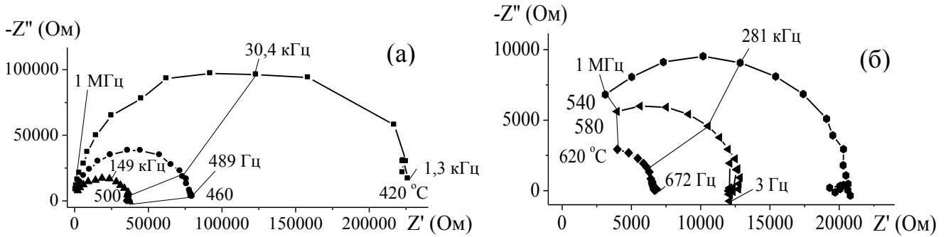
Рис. Г.7. Диаграммы импеданса (а, б) для \text{Bi}_{1,6}\text{Fe}_{0,42}\text{Ti}_2\text{O}_{7-\delta} , t (°C): 420; 460; 500; 540; 620.
