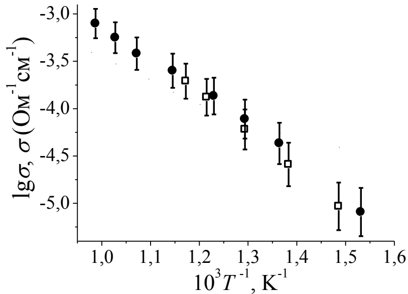
Рис. 7.5. Проводимость \text{Bi}_{1,6}\text{Fe}_{0,3}\text{Ti}_2\text{O}_{7-\delta} (указана погрешность 5 %), измеренная двухзондовым методом при 1 кГц (закрашенные кружки) и методом импедансной спектроскопии (квадраты) при \omega \rightarrow 0 .
