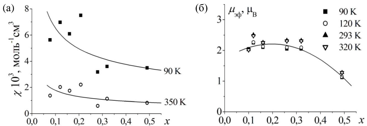
Рис. 6.17. Концентрационные и температурные зависимости \chi^{\text{пара}} (а) и \mu_{\text{эф}} меди в \text{Bi}_{1,6}\text{Cu}_x\text{Ti}_2\text{O}_{7-\delta} (б).
