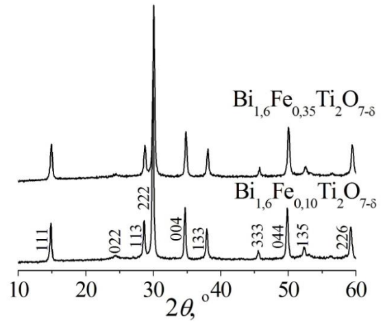
Рис. 3.4. Дифрактограммы \text{Bi}_{1,6}\text{Fe}_x\text{Ti}_2\text{O}_{7-\delta} ( x = 0,10; 0,35 , гидротермальный метод).
