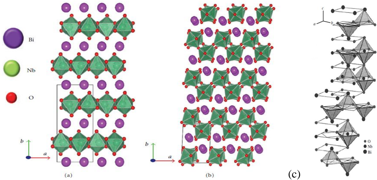
Рис. 1.2. Структуры \text{BiNbO}_4 [3]: (a) – ромбическая низкотемпературная; (b) – триклинная высокотемпературная; (c) – ромбическая \text{Bi}_5\text{Nb}_3\text{O}_{15} [4].
