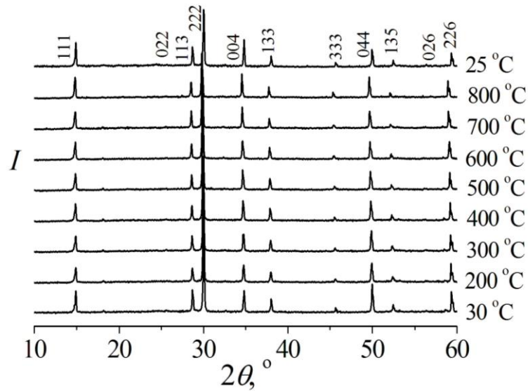
Рис. Б.4. Дифрактограммы \text{Bi}_{1,60}\text{Fe}_{0,42}\text{Ti}_2\text{O}_{7-\delta} ( Fd\bar{3}m ).
