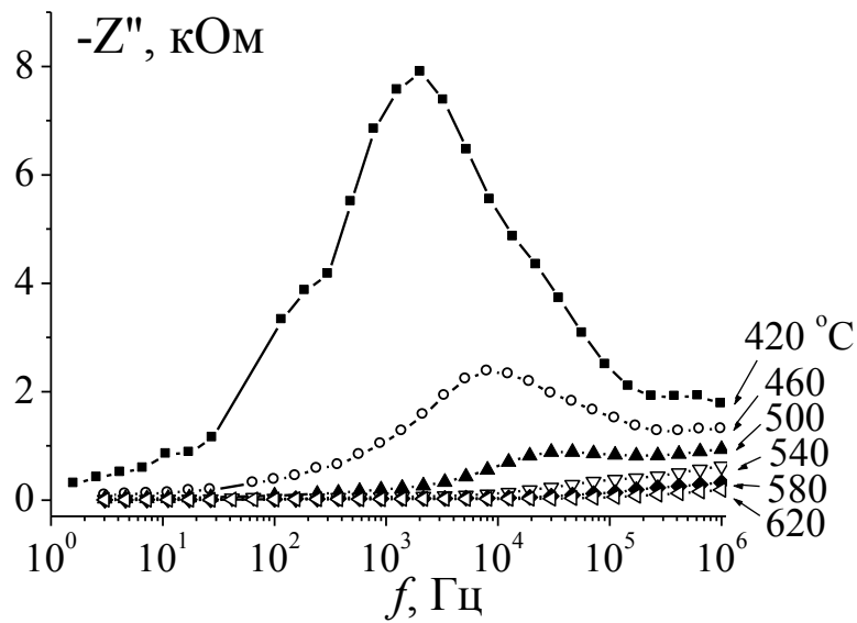
Рис. Г.6. Частотная зависимость мнимой части импеданса \text{Bi}_{1,6}\text{Fe}_{0,3}\text{Ti}_2\text{O}_{7-\delta} .
