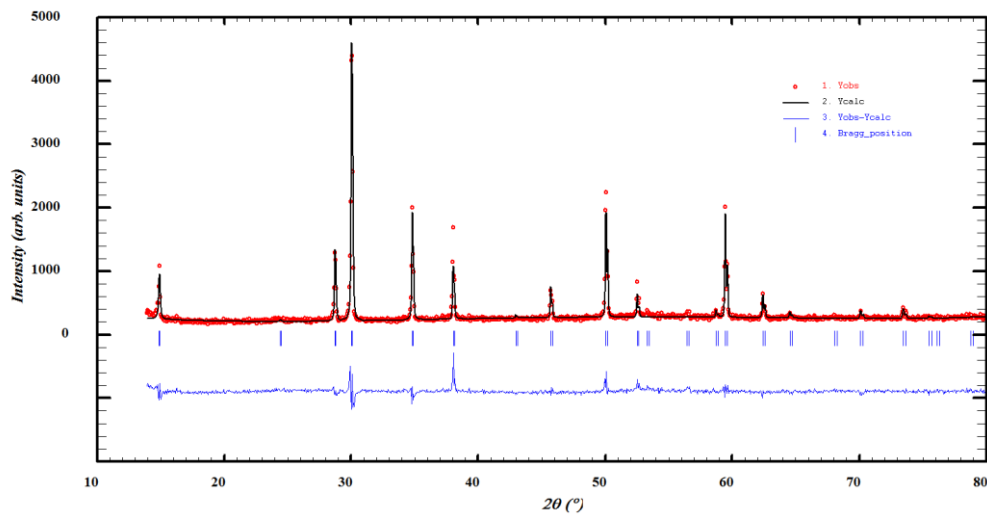
Рис. Б.6. Дифрактограмма \text{Bi}_{1,6}\text{Mn}_{0,5}\text{Ti}_2\text{O}_{7-\delta} ( \text{Bi}_{1,56}\text{Mn}_{0,44}\text{Ti}_{1,95}\text{Mn}_{0,05}\text{O}_{7-\delta} ).
