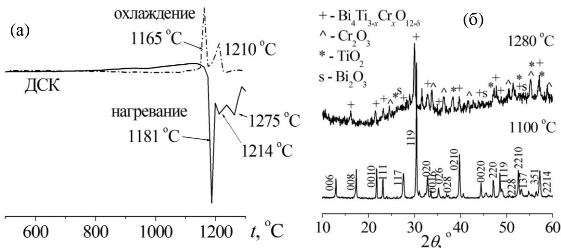
Рис. 3.16. (а) – Кривые ДСК для \text{Bi}_4\text{Ti}_{2,80}\text{Cr}_{0,20}\text{O}_{12-\delta} и (б) – дифрактограммы \text{Bi}_4\text{Ti}_{1,80}\text{Cr}_{1,19}\text{O}_{12-\delta} при 298 К до плавления и после кристаллизации.
