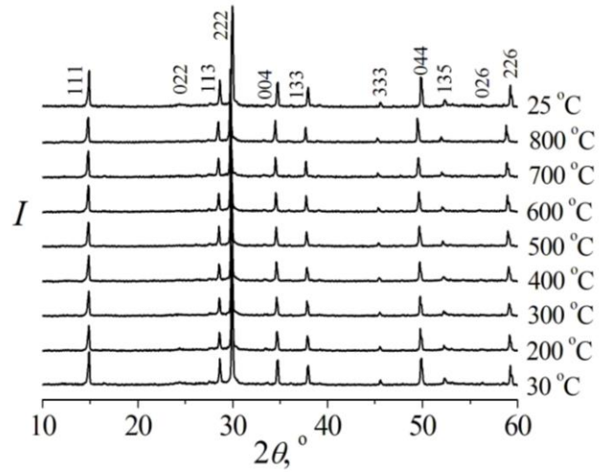
Рис. Б.3. Дифрактограммы \text{Bi}_{1,6}\text{Cr}_{0,20}\text{Ti}_2\text{O}_{7-\delta} ( Fd\bar{3}m ).
