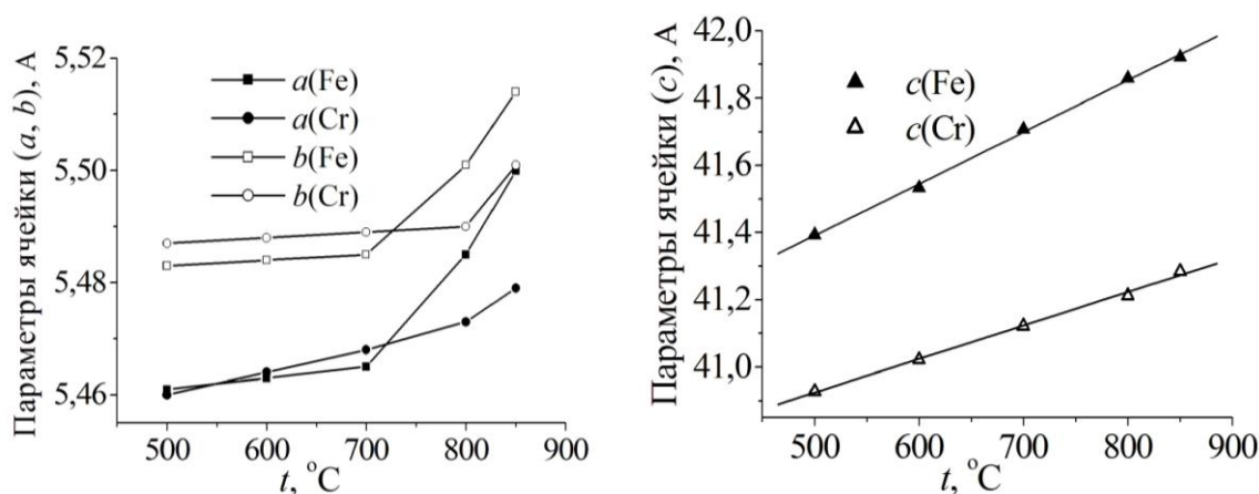
Рис. 4.10. Параметры \text{Vi}_4\text{Ti}_{1,5}\text{Cr}_{1,5}\text{O}_{11,25} и \text{Vi}_4\text{Ti}_{2,20}\text{Fe}_{0,88}\text{O}_{11,72} ( Fmm2 , m = 4 ) при 550 – 850 °С.
