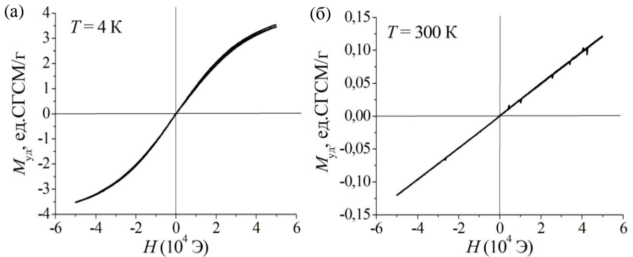
Рис. 6.10. Зависимость удельной намагниченности \text{Bi}_{1,6}\text{Ti}_2\text{Mn}_{0,1}\text{O}_{7-\delta} от поля при 4 (а) и 300 (б) К.
