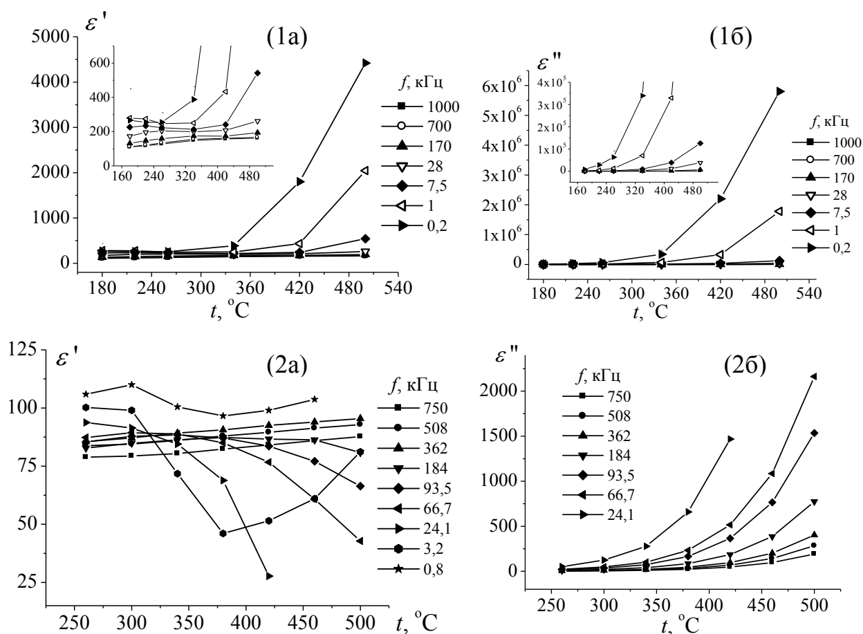
Рис. 7.16. Температурные зависимости действительной \epsilon' (а) и мнимой \epsilon'' (б) части диэлектрической проницаемости \text{Bi}_{1,6}\text{Mn}_{0,8}\text{Ti}_{1,6}\text{O}_{7-\delta} (1а,1б) и \text{Bi}_{1,86}\text{Mn}_{0,28}\text{Ti}_{1,86}\text{O}_{7-\delta} (2а ,2б) при разных частотах.
