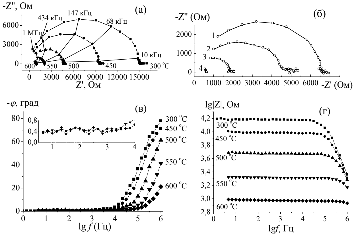
Рис. Г.11. Диаграммы импеданса на комплексной плоскости: \text{Bi}_{1,6}\text{Cu}_{0,2}\text{Ti}_2\text{O}_{7-\delta} (а) и \text{Bi}_{1,6}\text{Cu}_{0,8}\text{Ti}_2\text{O}_{7-\delta} (б, 1 – 300^\circ\text{C} ; 2 – 400^\circ\text{C} ; 3 – 500^\circ\text{C} ; 4 – 600^\circ\text{C} ) и диаграммы Боде для \text{Bi}_{1,6}\text{Cu}_{0,2}\text{Ti}_2\text{O}_{7-\delta} (в, г).
