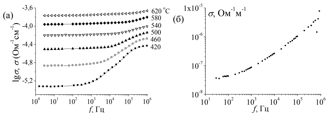
Рис. 7.21. Частотные зависимости проводимости (а) – \text{Bi}_{1,6}\text{Fe}_{0,3}\text{Ti}_2\text{O}_{7-\delta} при 420–620 °С и (б) – \text{Bi}_{1,6}\text{Cr}_{0,16}\text{Ti}_2\text{O}_{7-\delta} при 25 °С.
