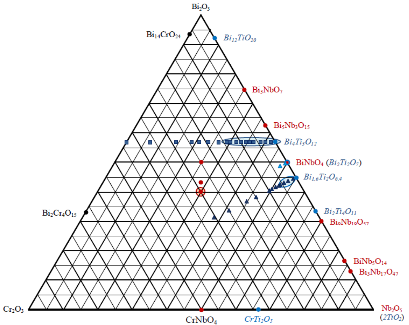
Рис. 3.8. Концентрационный треугольник для систем \text{Bi}_2\text{O}_3\text{--Cr}_2\text{O}_3\text{--Nb}_2\text{O}_5 [10] и \text{Bi}_2\text{O}_3\text{--Cr}_2\text{O}_3\text{--TiO}_2 .
