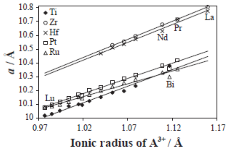
Рис. 1.10. Зависимости параметра ячейки (298 К) пирохлоров A_2B_2O_7 ( A – катионы редкоземельных элементов и висмута) от ионного радиуса A [79].
