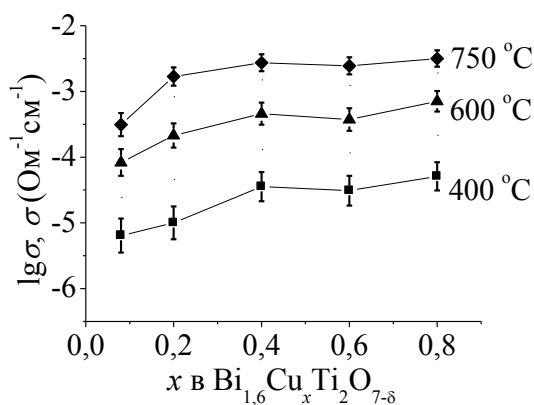
Рис. 7.23. Концентрационная зависимость проводимости \text{Bi}_{1.6}\text{Ti}_2\text{Cu}_x\text{O}_{7-\delta} (воздух, охлаждение, указана погрешность 5 %) при 400 – 750 °C.
