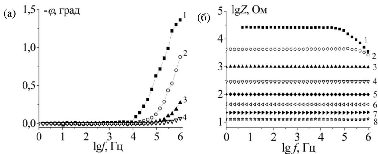
Рис. 7.7. Частотные зависимости фазового угла (а) и модуля импеданса (б) \text{Bi}_{1,33}\text{Mn}_{1,33}\text{Nb}_{1,33}\text{O}_{6,65} , измеренные при температурах ( ^\circ\text{C} ) 100(1), 150(2), 200(3), 250(4), 300(5), 350(6), 400(7), 450(8).
