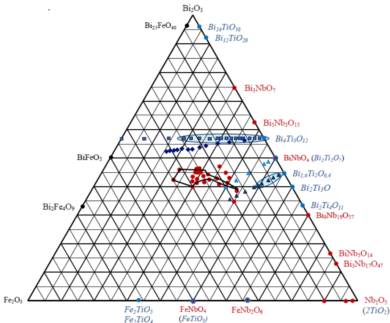
Рис. 3.9. Концентрационный треугольник для систем \text{Bi}_2\text{O}_3\text{--Fe}_2\text{O}_3\text{--Nb}_2\text{O}_5 [88] и \text{Bi}_2\text{O}_3\text{--Fe}_2\text{O}_3\text{--TiO}_2 .
