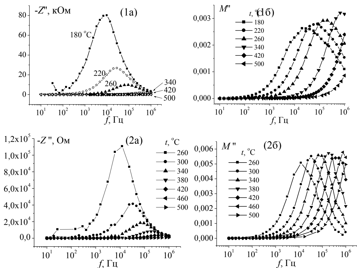
Рис. 7.18. Частотная зависимость мнимых частей импеданса Z'' (а) и электрического модуля M'' (б) при температурах 180-500 °С для \text{Bi}_{1,6}\text{Mn}_{0,8}\text{Ti}_{1,6}\text{O}_{7-\delta} (1а, 1б) и \text{Bi}_{1,86}\text{Mn}_{0,28}\text{Ti}_{1,86}\text{O}_{7-\delta} (2а, 2б).
