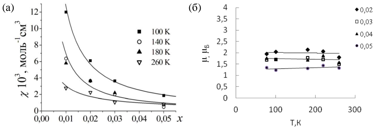
Рис. 6.20. Парамагнитная составляющая магнитной восприимчивости в зависимости от содержания меди ( x ) (а) и зависимость магнитного момента от температуры (б) для \text{Bi}_4\text{Ti}_{3-x}\text{Cu}_x\text{O}_{12-\delta} .
