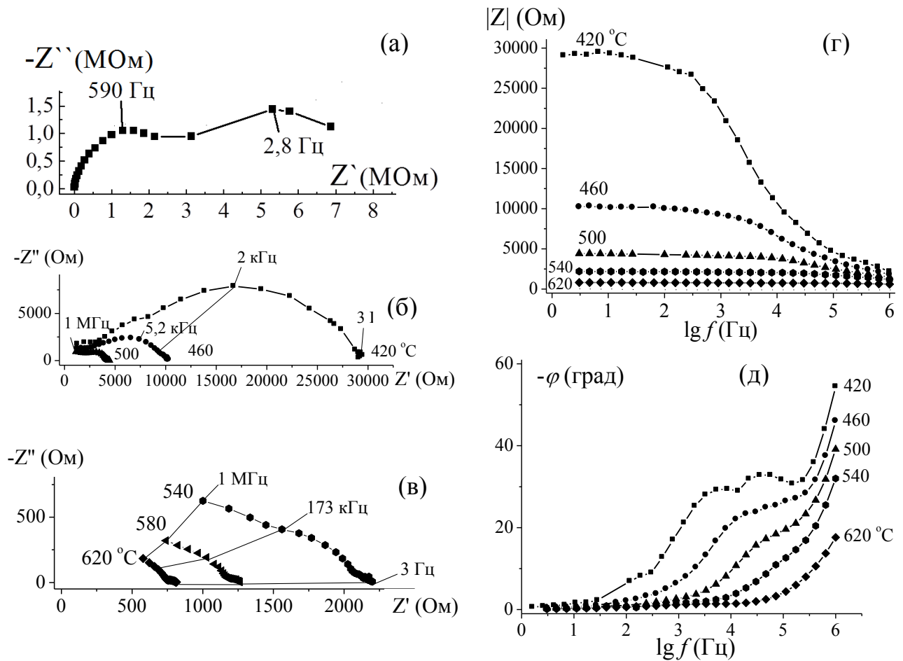
Рис. Г.3. Диаграммы импеданса на комплексной плоскости (а, б, в) и диаграммы Боде (г, д) для \text{Bi}_{1,6}\text{Fe}_{0,30}\text{Ti}_2\text{O}_{7-\delta} при t (°C): 23 (а); 420; 460; 500; 540; 620.
