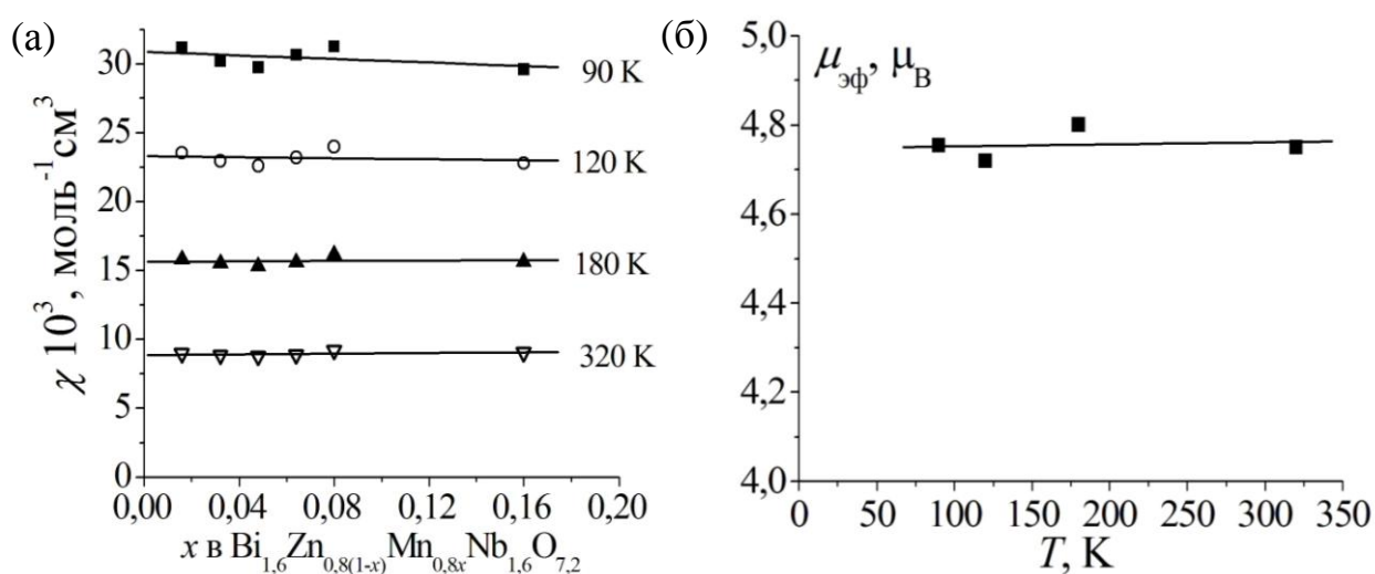
Рис. 6.12. Концентрационная зависимость парамагнитной составляющей магнитной восприимчивости (а) и температурные зависимости магнитного момента атома марганца для Bi_2Zn_{1-x}Mn_xNb_2O_{7-\delta} ( Bi_{1,6}Zn_{0,8-x}Mn_xNb_{1,6}O_{7,2} ) на бесконечном разбавлении ( x \rightarrow 0 ) (б).
