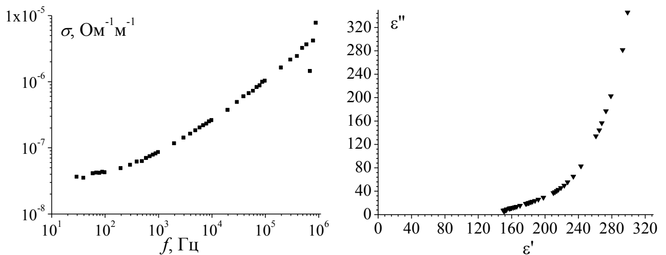
Рис. Г.12. Зависимости \sigma(f) и \varepsilon''(\varepsilon') для \text{V}_{1,6}\text{Cu}_{0,8}\text{Ti}_2\text{O}_{7-\delta} при 290 К.
