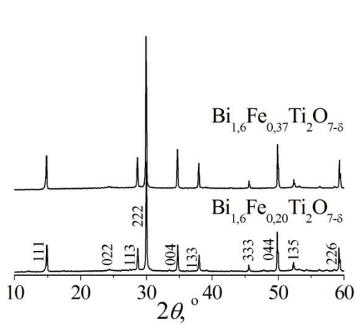
Рис. 3.3 Дифрактограммы \text{Bi}_{1,6}\text{Fe}_x\text{Ti}_2\text{O}_{7-\delta} ( x = 0,20; 0,37 , метод Печини).
