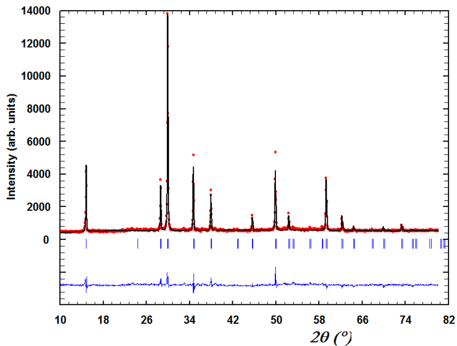
Рис. 4.4. Дифрактограмма для (\text{Bi}_{1,3}\text{Cu}_{0,31})(\text{Cu}_{0,31}\text{Ti}_{1,7})\text{O}_{7-\delta} .
