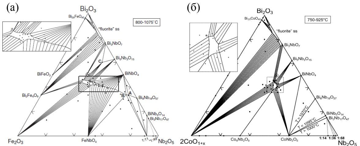
Рис. 1.12. Фазовый треугольник и «поле пироклора» в системе (а) \text{Bi}_2\text{O}_3\text{--Fe}_2\text{O}_3\text{--Nb}_2\text{O}_5 [88] и (б) \text{Bi}_2\text{O}_3\text{--}2\text{CoO}_{1+x}\text{--Nb}_2\text{O}_5 [89].
