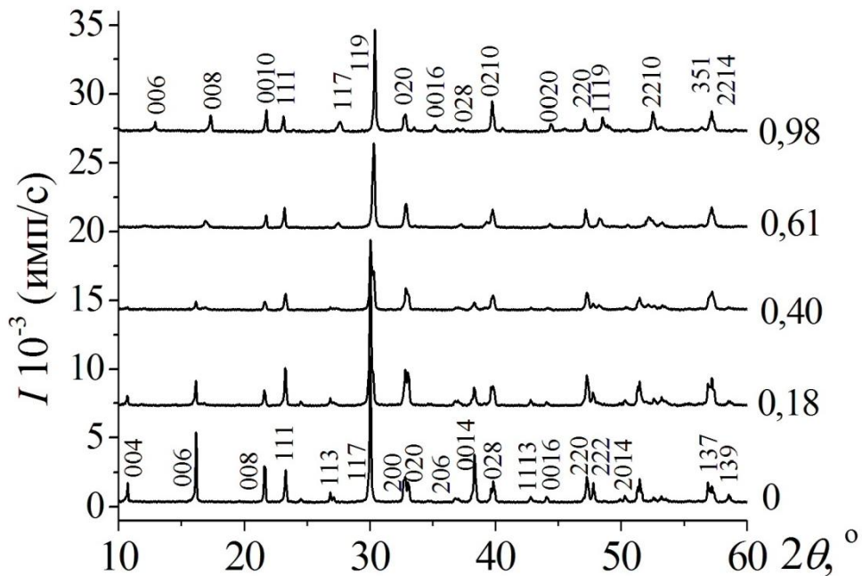
Рис. 3.5. Дифрактограммы \text{Bi}_4\text{Ti}_{3-x}\text{Cr}_x\text{O}_{12-\delta} .
