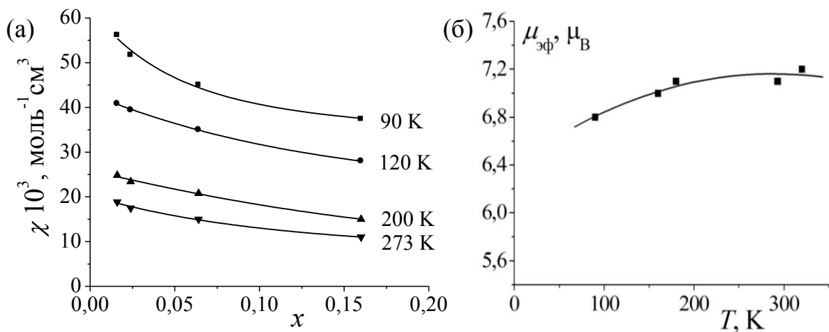
Рис. 6.8. Концентрационная зависимость магнитной восприимчивости (а) и температурная зависимость магнитного момента марганца для \text{Bi}_2\text{Mn}_x\text{Ti}_2\text{O}_{7-\delta} на бесконечном разбавлении ( x \rightarrow 0 ) (б).
