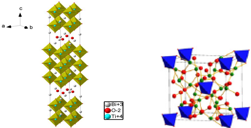
(a) \text{Bi}_4\text{Ti}_3\text{O}_{12} ( Fmmm ) [25]
