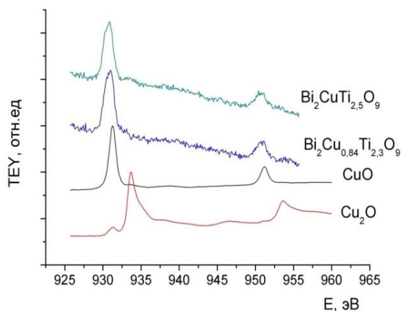
Рис. 5.5. NEXAFS Cu2p-спектров медьсодержащих титанатов висмута (пирохлоров) и оксидов меди [156].
