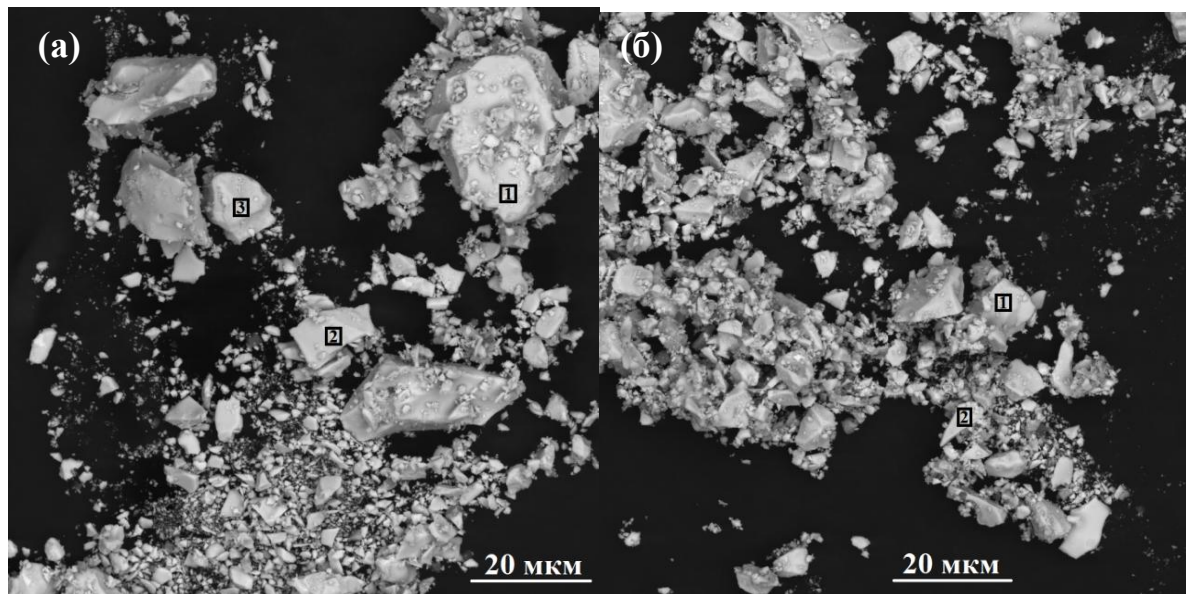
Рисунок А.1. СЭМ (а) \text{Bi}_{1,60}\text{Cu}_{0,20}\text{Ti}_2\text{O}_{7-\delta} (локальный энергодисперсионный анализ 1 – \text{Bi}_{1,69}\text{Cu}_{0,18}\text{Ti}_2\text{O}_{7-\delta} , 2 – \text{Bi}_{1,70}\text{Cu}_{0,20}\text{Ti}_2\text{O}_{7-\delta} , 3 – \text{Bi}_{1,69}\text{Cu}_{0,19}\text{Ti}_2\text{O}_{7-\delta} ) и (б) \text{Bi}_{1,60}\text{Cu}_{0,40}\text{Ti}_2\text{O}_{7-\delta} (1 – \text{Bi}_{1,74}\text{Cu}_{0,39}\text{Ti}_2\text{O}_{7-\delta} , 2 – \text{Bi}_{1,72}\text{Cu}_{0,30}\text{Ti}_2\text{O}_{7-\delta} ).
