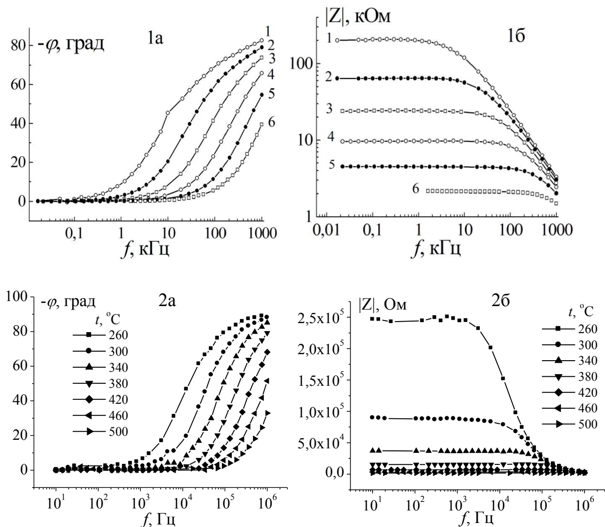
Рис. 7.13. Частотная зависимость (а) – фазового угла и (б) – модуля импеданса для \text{Bi}_{1,6}\text{Mn}_{0,8}\text{Ti}_{1,6}\text{O}_{6,4} (1а, 1б) при t (°C) 180 (1), 220 (2), 260 (3), 300 (4), 340 (5) и 380 (6) и для \text{Bi}_{1,86}\text{Mn}_{0,28}\text{Ti}_{1,86}\text{O}_{7-\delta} (2а,2б).
