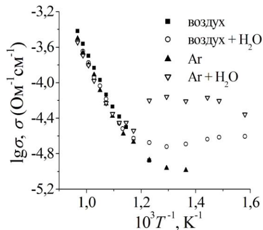
Рис. 7.29. Проводимость Vi_{1,6}Fe_{0,30}Ti_2O_{7-8} в разных средах.
