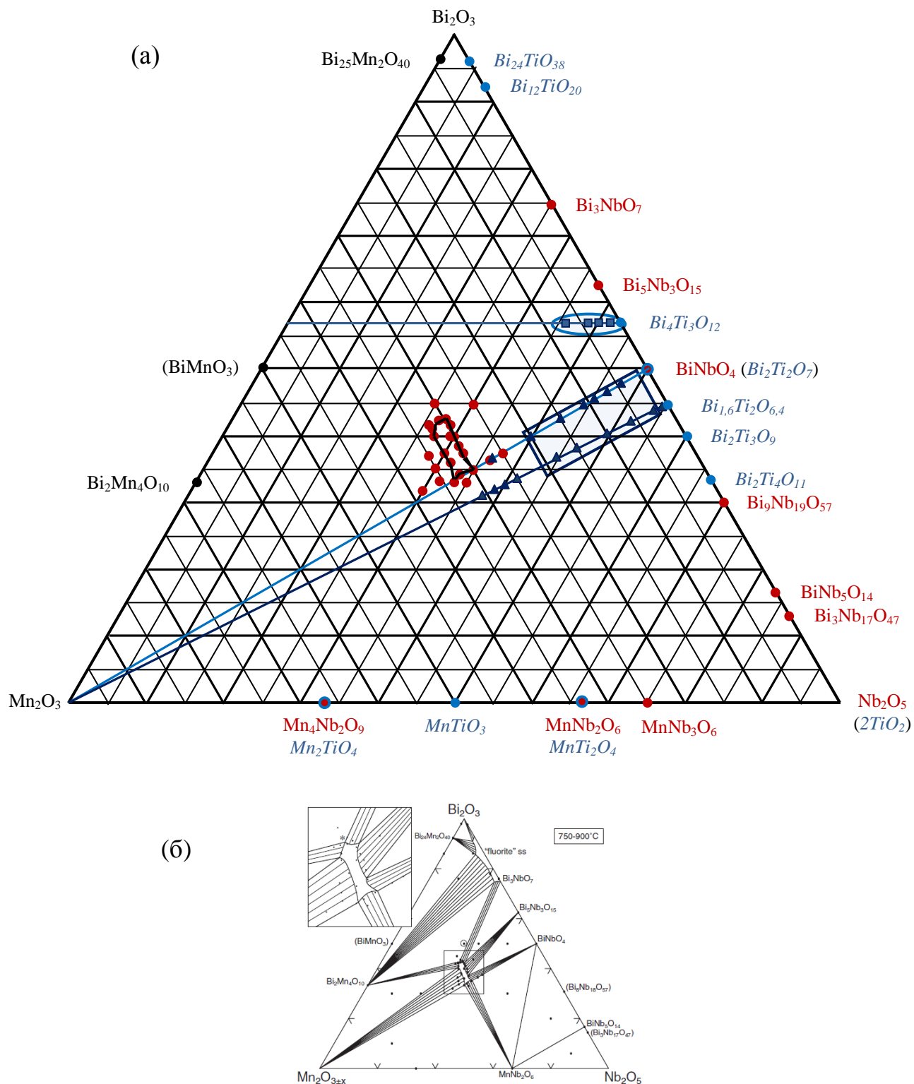
Рис. 3.10. Фигуративные точки составов, соответствующие допированным марганцем титанатам висмута на концентрационном треугольнике (а). Знаками в виде затушеванных треугольников обозначены соединения со структурой пироклора, знаками в виде квадратов – составы со слоистой структурой; (б) – фазовый треугольник в системе \text{Bi}_2\text{O}_3\text{-Mn}_2\text{O}_3\text{-Nb}_2\text{O}_5 [87] с выделенной областью пироклоров.
