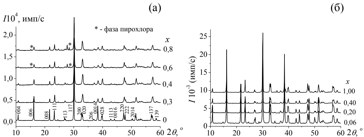
Рис. 3.7. Дифрактограммы \text{Bi}_4\text{Ti}_{3-x}\text{Mn}_x\text{O}_{12-\delta} (а) и \text{Bi}_4\text{Ti}_{3-x}\text{Cu}_x\text{O}_{12-\delta} x \leq 0,6 (б).
