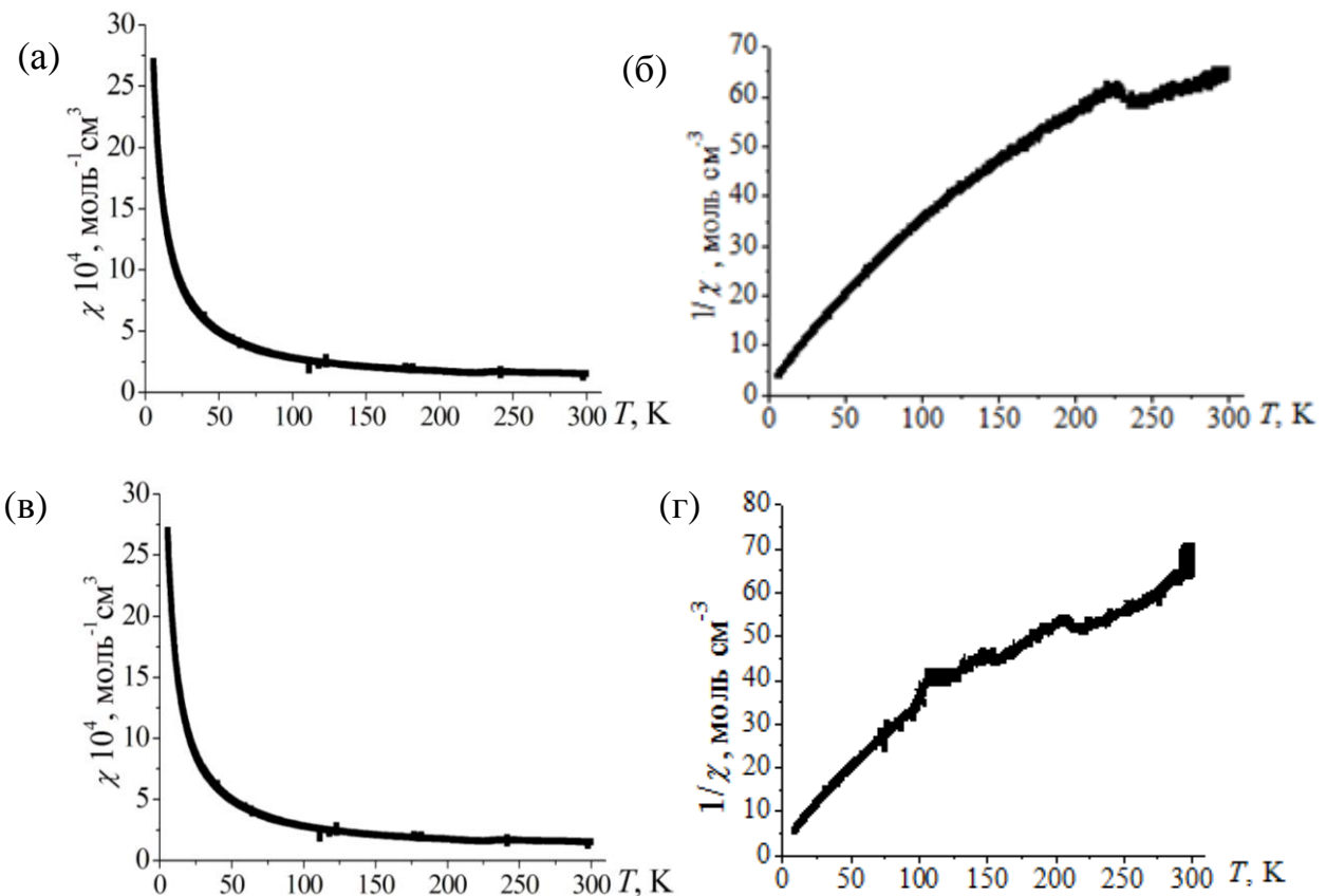
Рис. 6.15. Температурная зависимость магнитной восприимчивости (а, в) и ее обратной величины (б, г) для \text{Bi}_4\text{Ti}_{2,95}\text{Mn}_{0,05}\text{O}_{12-\delta} при 3 (а, б) и 5 (в, г) Тл.
