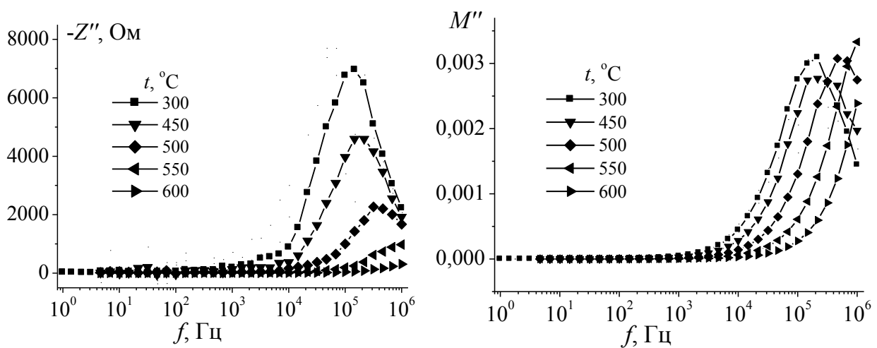
Рис. 7.25. Частотная зависимость мнимых частей импеданса Z'' (а) и электрического модуля M'' (б) при температурах 300-600 °С для \text{Bi}_{1,6}\text{Cu}_{0,2}\text{Ti}_2\text{O}_{7-\delta}
