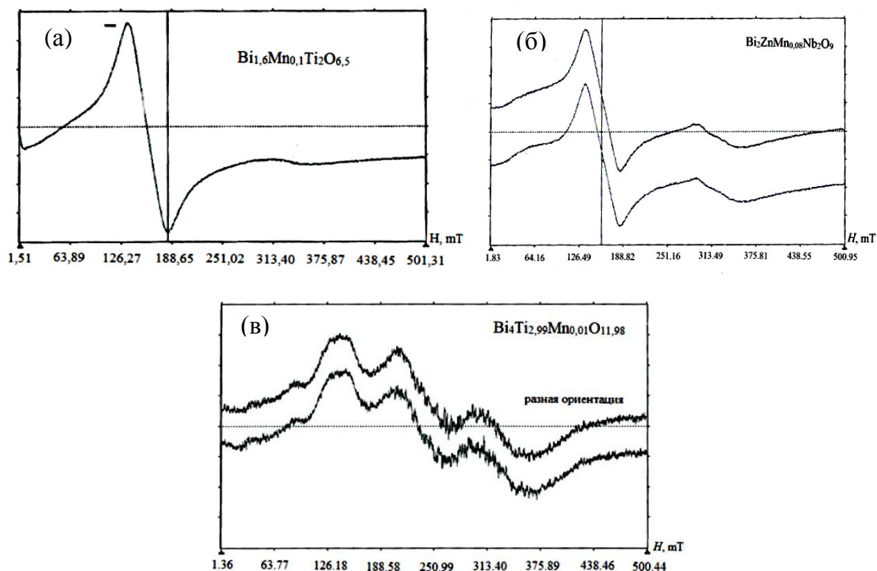
Рис. 5.13. ЭПР спектры \text{Bi}_{1,6}\text{Mn}_{0,1}\text{Ti}_2\text{O}_{6,5} (а), \text{Bi}_{1,6}\text{Zn}_{0,92}\text{Mn}_{0,08}\text{Nb}_2\text{O}_7 (б), \text{Bi}_4\text{Mn}_{0,01}\text{Ti}_{2,99}\text{O}_{7-\delta} (в) при комнатной температуре.
