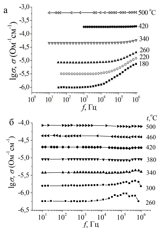
Рис. 7.15. Частотная зависимость проводимости для \text{Bi}_{1,6}\text{Mn}_{0,8}\text{Ti}_{1,6}\text{O}_{7-\delta} (а) и \text{Bi}_{1,86}\text{Mn}_{0,28}\text{Ti}_{1,86}\text{O}_{7-\delta} (б) при указанных температурах.
