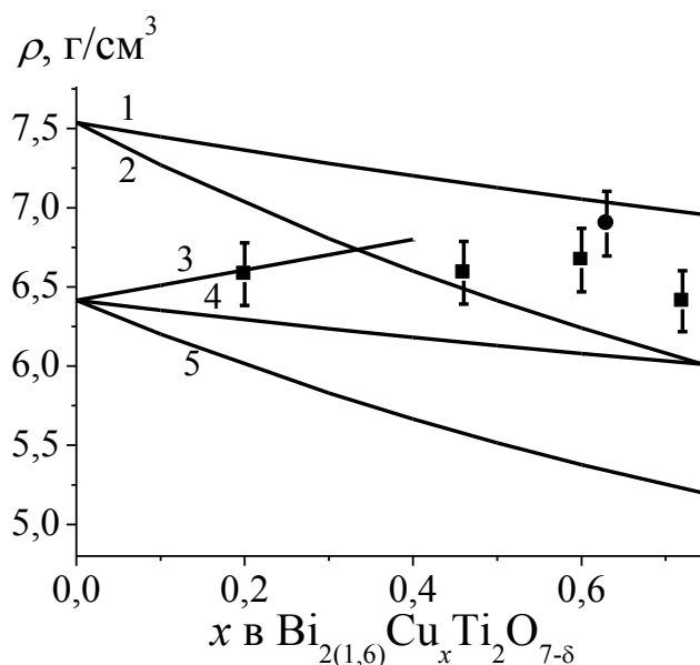
Рис. 4.8. Зависимость плотности пикнометрической и рентгенографической для a = 10,330 \text{ \AA} и разного распределения меди по катионным позициям от общего содержания меди. Пронумерованные графики соответствуют следующим моделям распределения:
