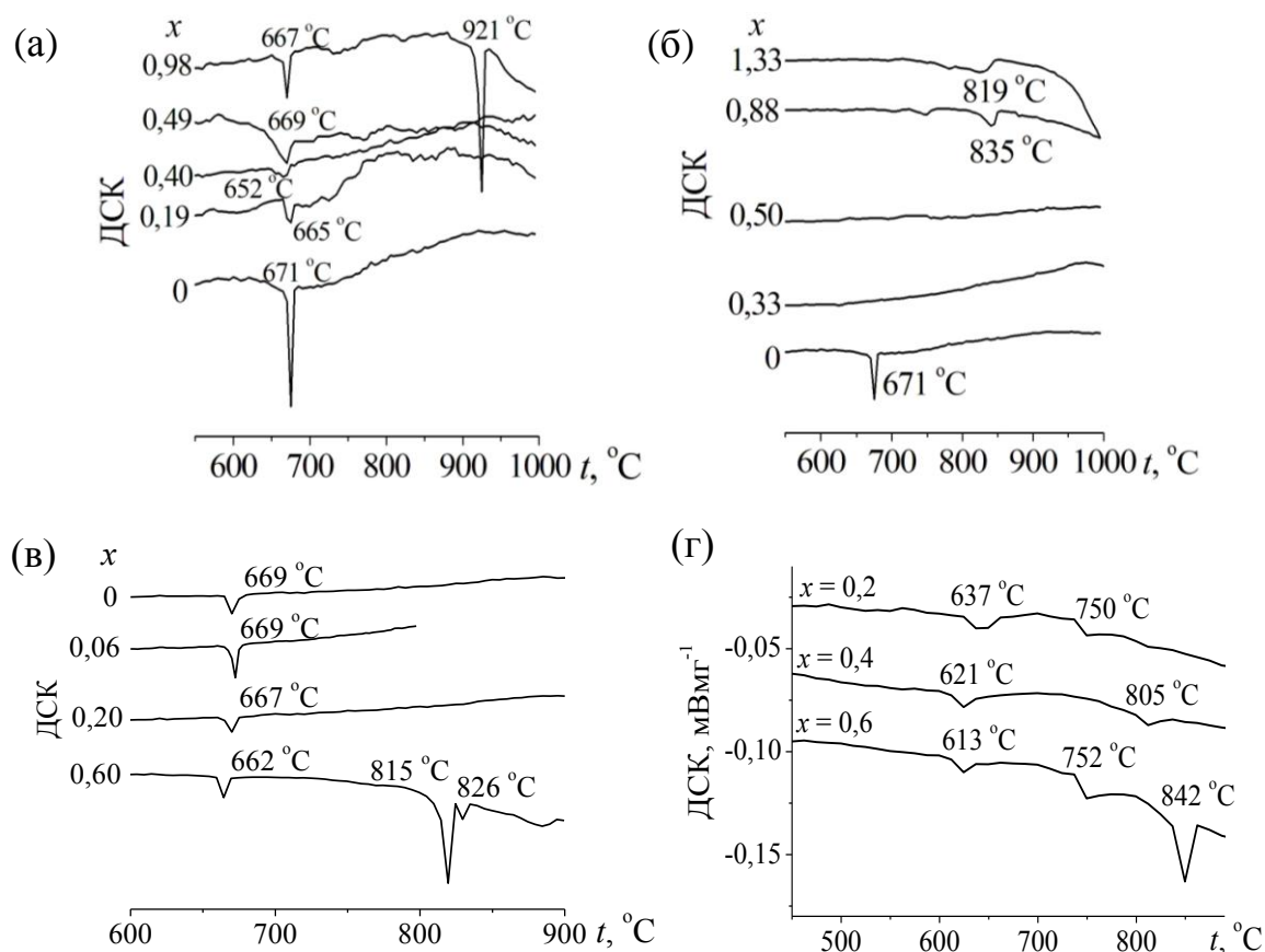
Рис. 4.11. ДСК (нагревание) образцов \text{Bi}_4\text{Ti}_{3-x}\text{Cr}_x\text{O}_{12-\delta} (а), \text{Bi}_4\text{Ti}_{3-x}\text{Fe}_x\text{O}_{12-\delta} (б), \text{Bi}_4\text{Ti}_{3-x}\text{Cu}_x\text{O}_{12-\delta} (в), \text{Bi}_4\text{Ti}_{3-x}\text{Mn}_x\text{O}_{12-\delta} (г).
