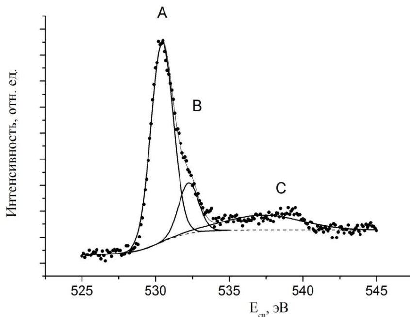
Рис. 5.10. XPS-спектр кислорода в \text{Bi}_{1,9}\text{Mn}_{0,2}\text{Ti}_{1,9}\text{O}_{6,9} .
