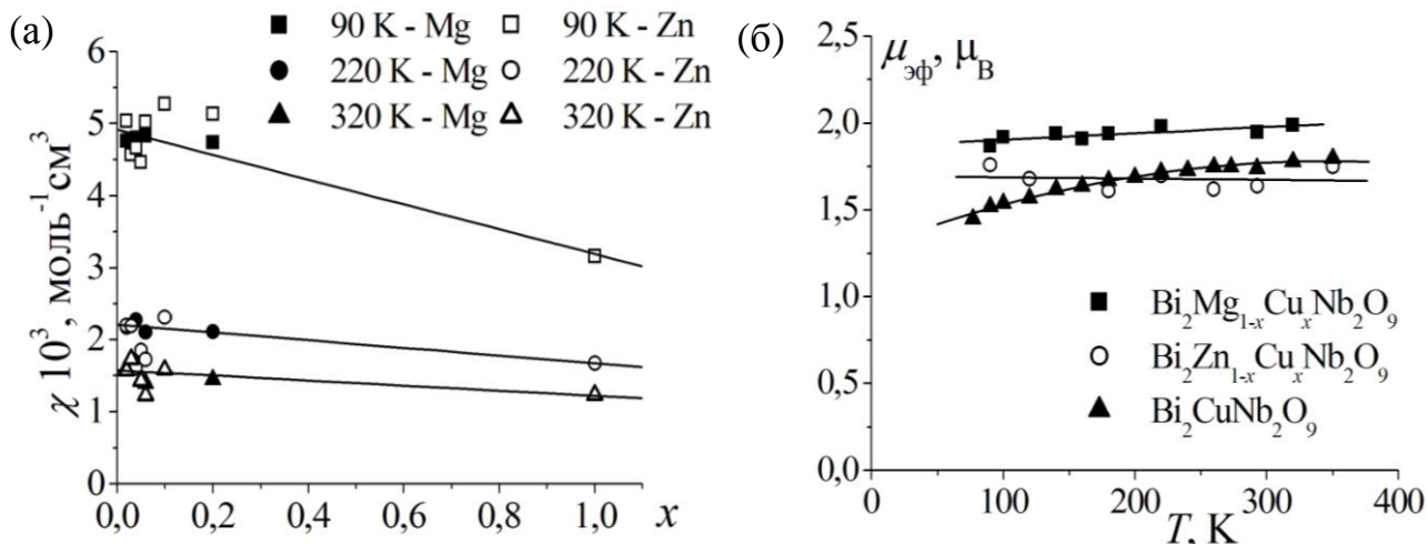
Рис. 6.19. Концентрационные и температурные зависимости магнитной восприимчивости (а) и эффективного магнитного момента меди (б) для \text{Bi}_2\text{CuNb}_2\text{O}_9 ( \text{Bi}_{1,6}\text{Cu}_{0,8}\text{Nb}_{1,6}\text{O}_{7-\delta} ) и экстраполированных на предельное разбавление \mu_{\text{эф}}(x \rightarrow 0) \text{Bi}_2\text{Mg}_{1-x}\text{Cu}_x\text{Nb}_2\text{O}_{7-\delta} ( \text{Bi}_{1,6}\text{Mg}_{0,8-0,8x}\text{Cu}_{0,8x}\text{Nb}_{1,6}\text{O}_{7-\delta} ) и \text{Bi}_2\text{Zn}_{1-x}\text{Cu}_x\text{Nb}_2\text{O}_{7-\delta} ( \text{Bi}_{1,6}\text{Zn}_{0,8-0,8x}\text{Cu}_{0,8x}\text{Nb}_{1,6}\text{O}_{7-\delta} ).
