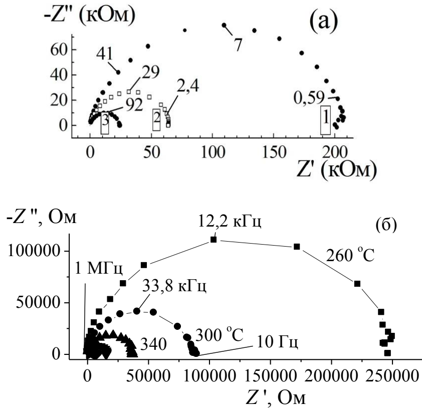
Рис. 7.12. Диаграммы импеданса: (а) – \text{Bi}_{1,6}\text{Mn}_{0,8}\text{Ti}_{1,6}\text{O}_{7-\delta} при t ( ^{\circ}\text{C} ): 180 (1); 220 (2) и 260 (3); частота в (кГц) указана в виде цифр при выделенных точках (б) – \text{Bi}_{1,86}\text{Mn}_{0,28}\text{Ti}_{1,86}\text{O}_{7-\delta} .
