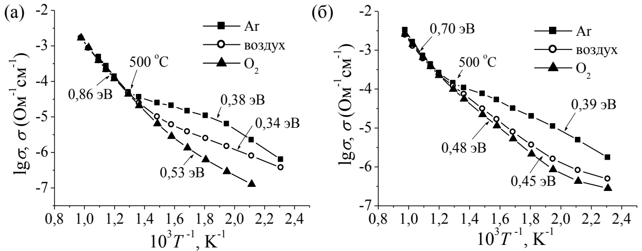
Рис. 7.24. Температурные зависимости проводимости \text{Bi}_{1.6}\text{Cu}_{0.2}\text{Ti}_2\text{O}_{7-\delta} (а), \text{Bi}_{1.6}\text{Cu}_{0.6}\text{Ti}_2\text{O}_{7-\delta} (б).
