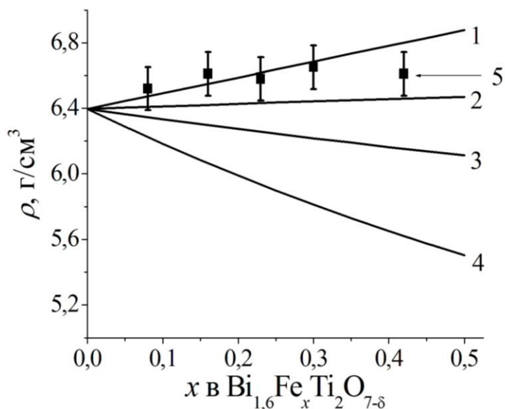
Рис. 4.6. Зависимости пикнометрической и рентгенографической ( a = 10,345 \text{ \AA} ) плотностей пироксенов с разным распределением железа по катионным подрешеткам от общего содержания железа. Пронумерованные графики соответствуют следующим моделям распределения: 1 – (\text{Bi}_{1,6}\text{Fe}_x)\text{Ti}_2\text{O}_{7-\delta} , 2 – (\text{Bi}_{3,2/(2+x/4)}\text{Fe}_{3x/4})(\text{Fe}_{x/4}\text{Ti}_2)\text{O}_{7-\delta} , 3 – (\text{Bi}_{3,2/(2+x/2)}\text{Fe}_{x/2})(\text{Fe}_{x/2}\text{Ti}_2)\text{O}_{7-\delta} , 4 – \text{Bi}_{3,2/(2+x)}(\text{Ti}_2\text{Fe}_x)\text{O}_{7-\delta} , 5 – \rho_{\text{пикн}} .
