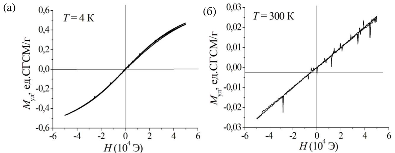
Рис. 6.16. Зависимость намагниченности (а, б) \text{V}_4\text{Ti}_{2,95}\text{Mn}_{0,05}\text{O}_{12-\delta} от напряженности магнитного поля при 4 (а) и 300 К (б).
