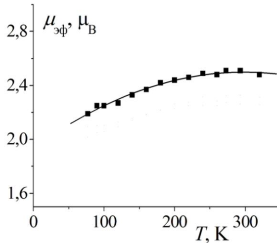
Рис.6.18 Температурная зависимость \mu_{\text{эф}} меди в \text{Bi}_{1,6}\text{Cu}_x\text{Ti}_2\text{O}_{7-\delta} при бесконечном разбавлении ( x \rightarrow 0 ).
