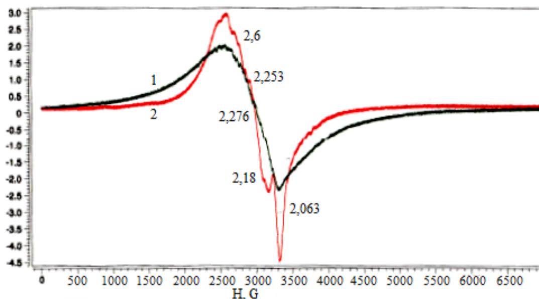
Рис. 5.14. ЭПР спектры порошков 1 – \text{Bi}_{1,6}\text{Cu}_{0,08}\text{Ti}_2\text{O}_{7-\delta} ; 2 – \text{Bi}_4\text{Cu}_{0,05}\text{Ti}_{2,95}\text{O}_{12-\delta} при комнатной температуре, g -фактор в обоих соединениях близок 2,25-2,28.
