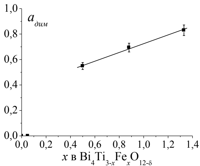
Рис. 6.6. Доля димеров \text{Fe}^{3+}\text{-O-Fe}^{3+} (90-293 К, J = -30 \text{ см}^{-1} ) в \text{Bi}_4\text{Ti}_{3-x}\text{Fe}_x\text{O}_{12-\delta} .
