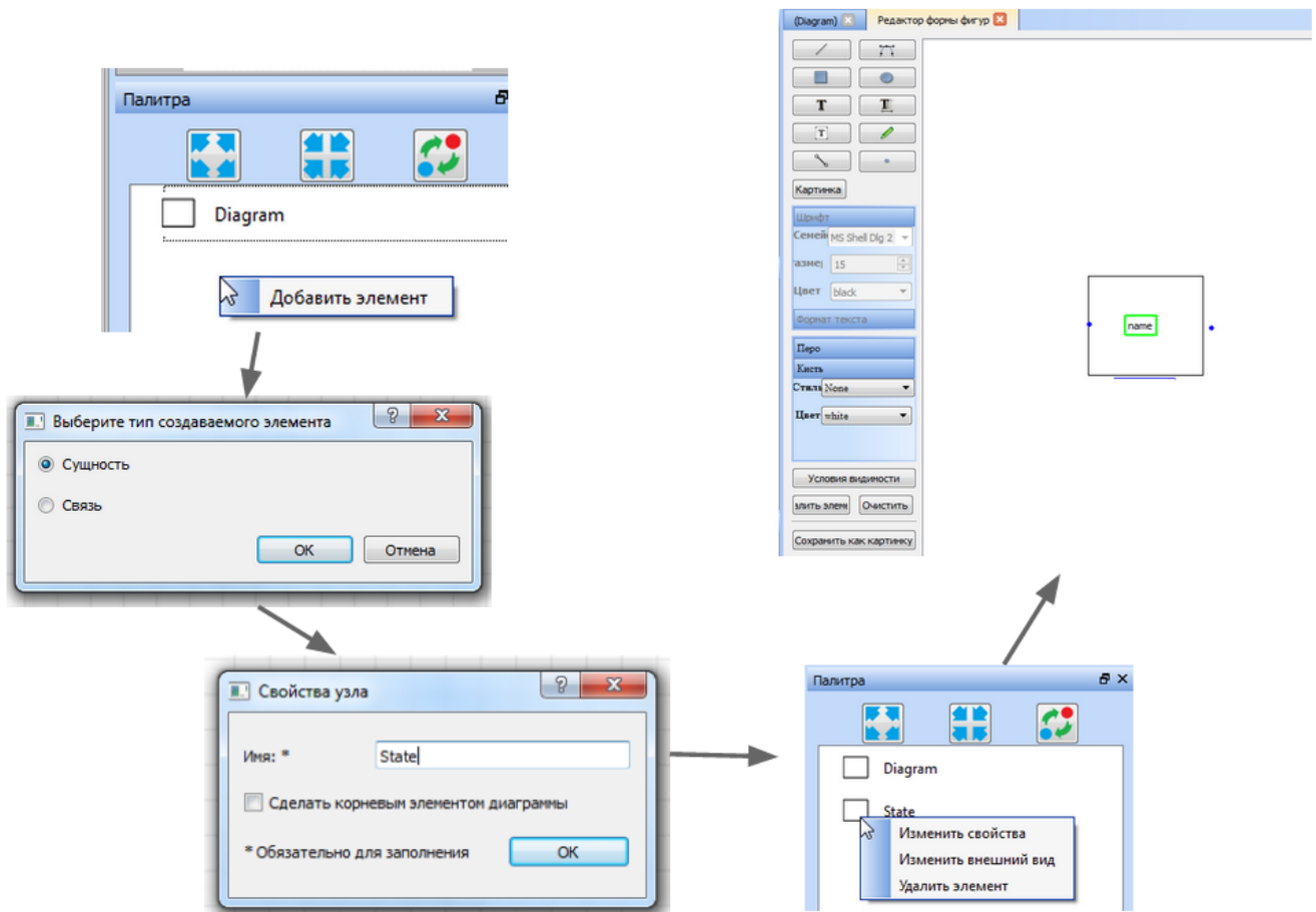
Рис. 4.7: Создание нового элемента языка.
