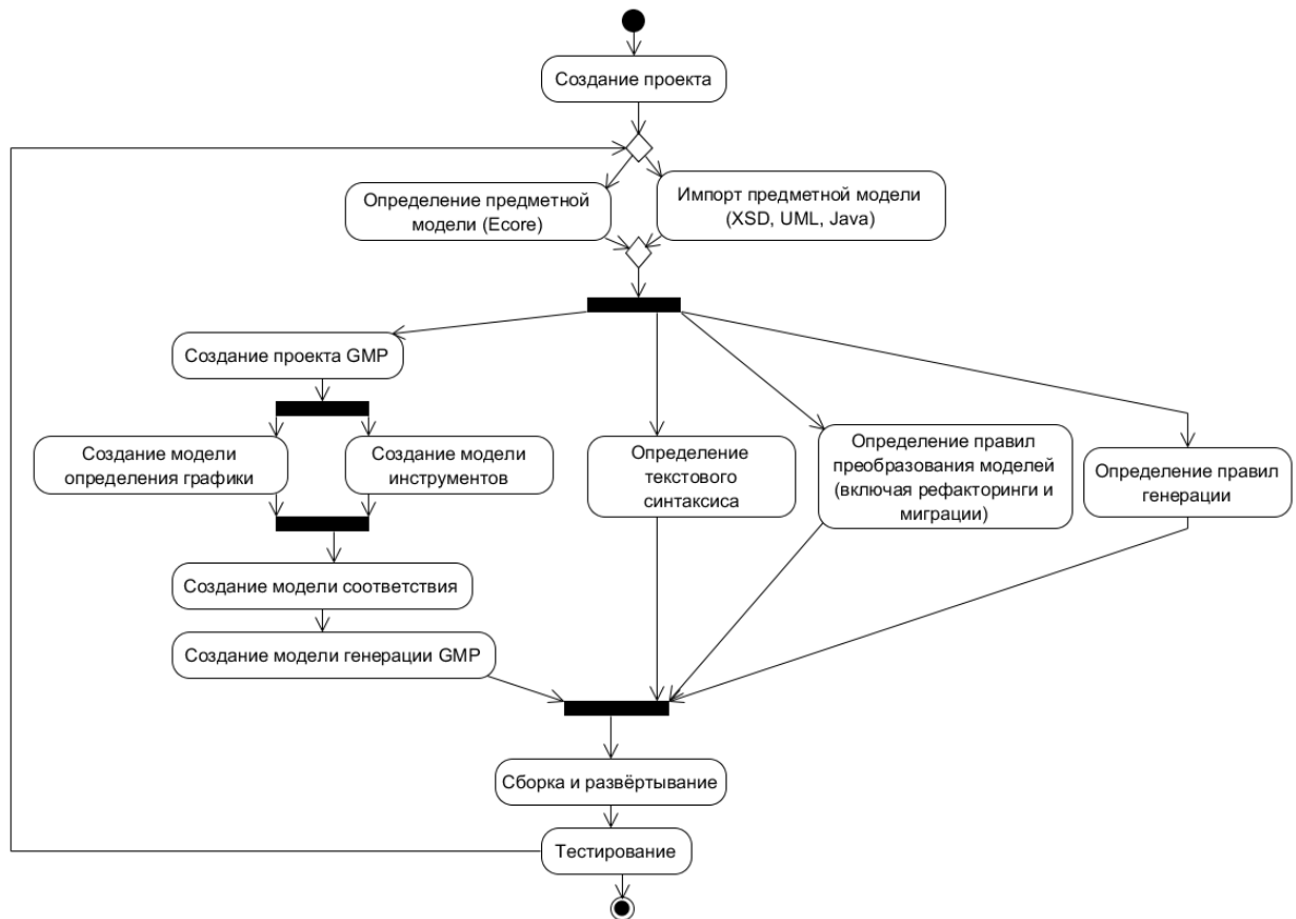
Рис. 2.2: Процесс создания DSM-решения на EMP.
