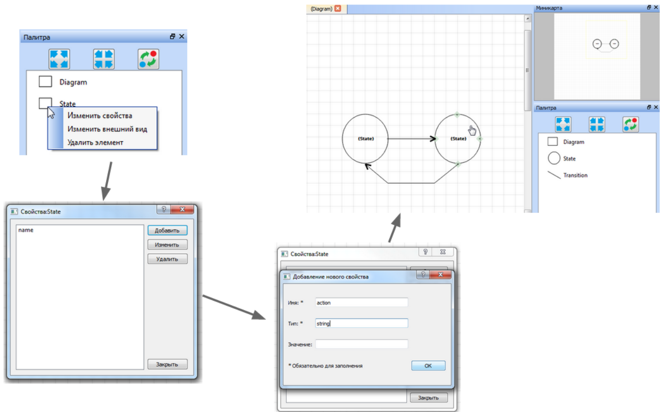
Рис. 4.8: Редактирование свойств элемента.
