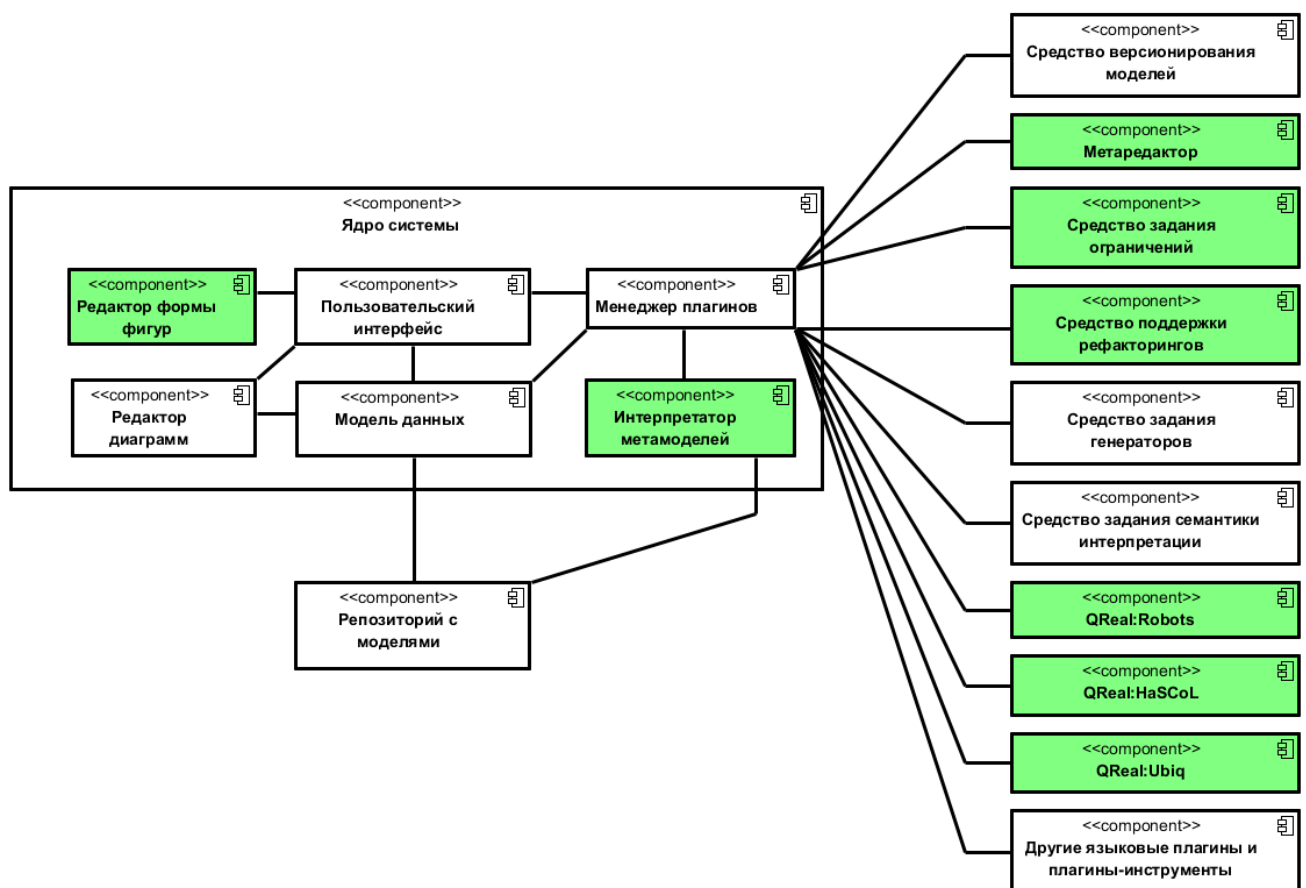
Рис. 4.1: Общая архитектура системы QReal.
