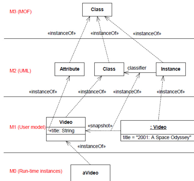
Рис. 2.1: Иерархия метаописаний UML, из [92].
