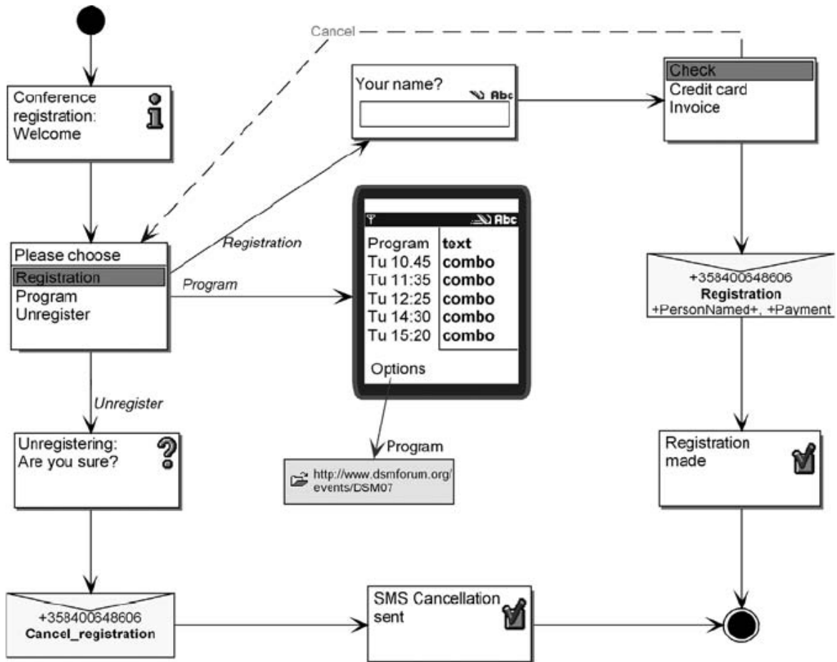
Рис. 1.2: Пример визуального предметно-ориентированного языка (рисунок из [36])
