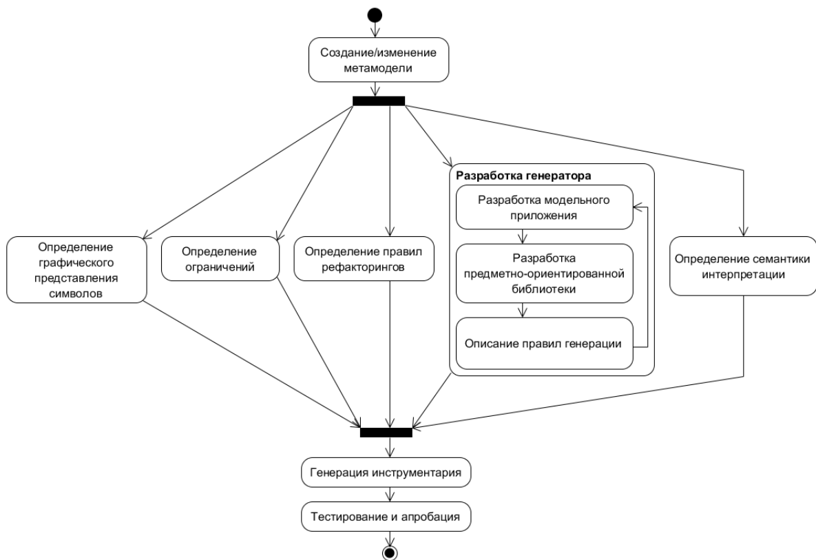
Рис. 3.2: Итерация проектирования и разработки языка.
