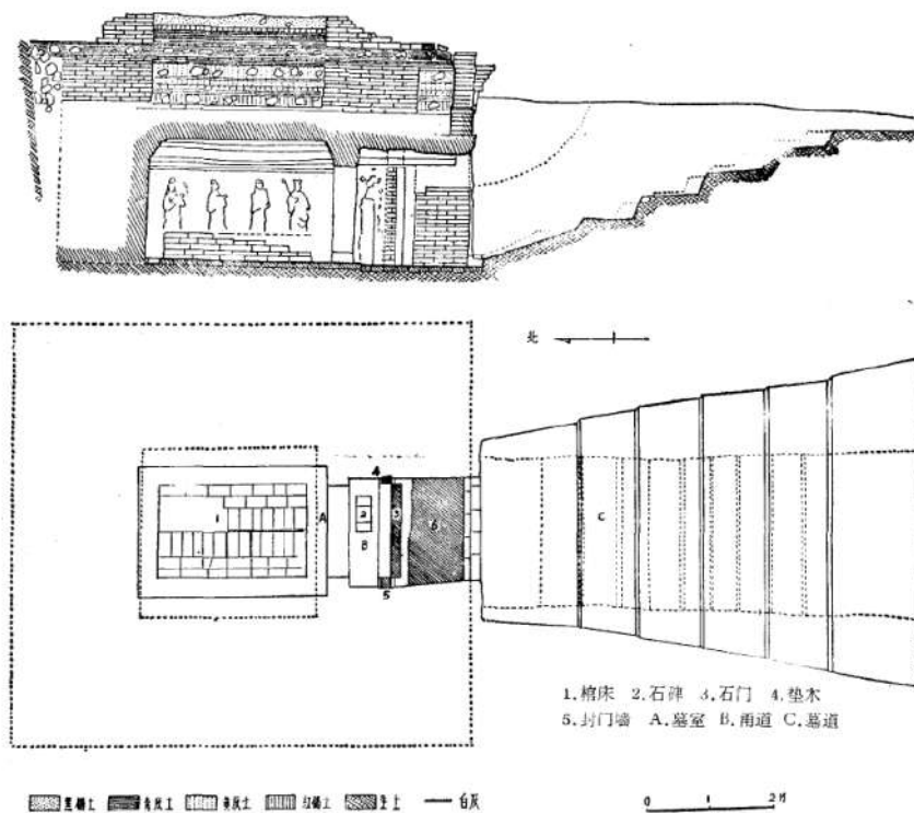
Рисунок 2.3.2.1 – План и профиль гробницы (могильной пагоды) принцессы Чжэньсяо. По: Яньбянь-Корейский автономный окружной музей, 1982, с. 176.
