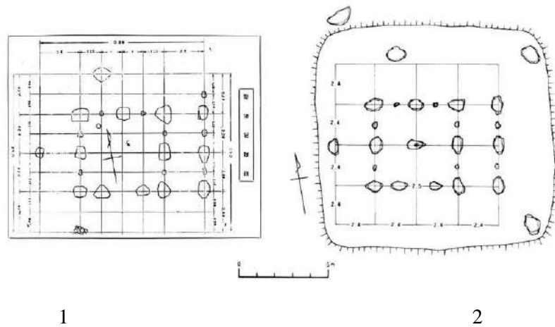
Рисунок 2.3.2.6 – Планировки Северо-восточного храма Балянчэн 1 – По: Торияма Киити, Фудзита Рёсаку, 1942, илл. 54; 2 – По: Сайто Ю, 1978, илл. 10.
